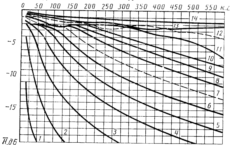
Значения параметра взаимности \bar{H} для ПЭП с круглой пьезопластиной, нагруженного на сталь 45
