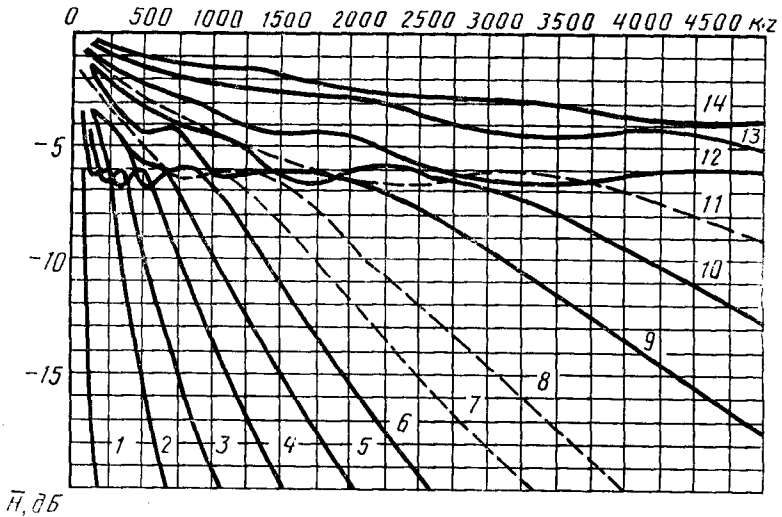
Значения параметра взаимности \bar{H} для ПЭП с квадратной пьезопластиной, нагруженного на воду
