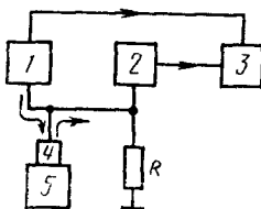
1—генератор видеоимпульсов; 2—широкополосный усилитель; 3—осциллограф; 4—проверяемый ПЭП; 5—акустическая нагрузка; R—резистор сопротивлением (50 \pm \pm 1) \text{ Ом}
