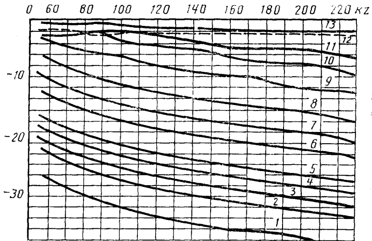
Значения параметра взаимности \bar{H} для ПЭП с круглой пьезопластиной, нагруженного на органическое стекло
