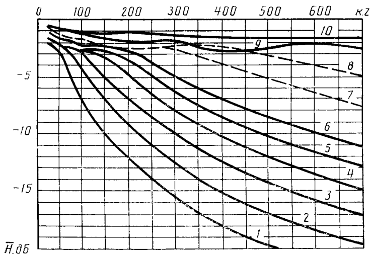
Значения параметра взаимности \bar{H} для ПЭП с круглой пьезопластиной, нагруженного на алюминиевый сплав Д16Т
