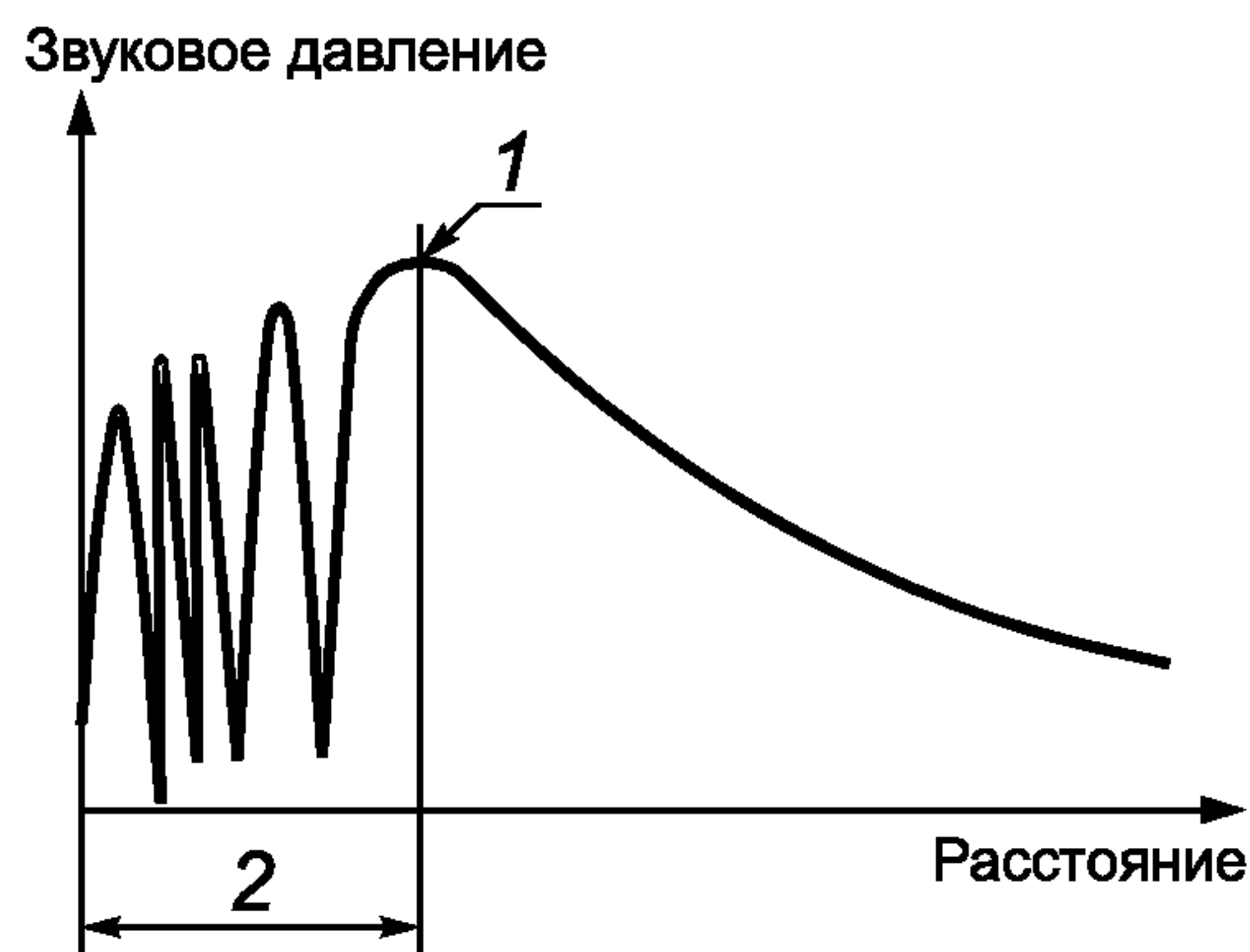
1 — граница ближней зоны (2.1.20); 2 — протяженность ближней зоны (2.1.19)
