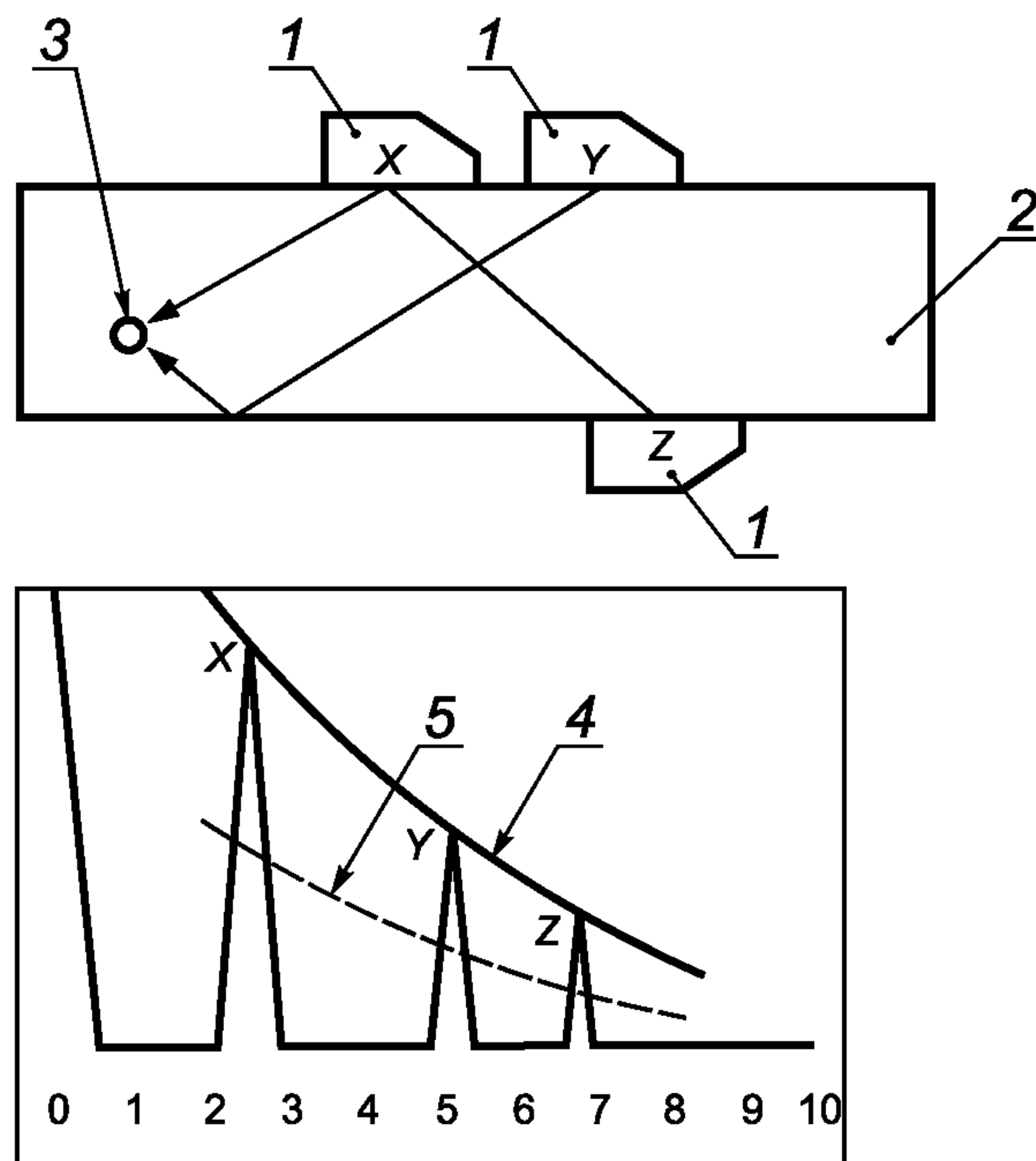
1 — наклонный преобразователь (2.5.1); 2 — контрольный образец (2.7.3); 3 — контрольный отражатель (2.7.4), боковой цилиндрический отражатель (2.7.5); 4 — кривая коррективки амплитуда-расстояние (АРК-кривая) (2.12.4); 5 — уровень 50 % АРК-кривой; X, Y, Z — положение преобразователя
