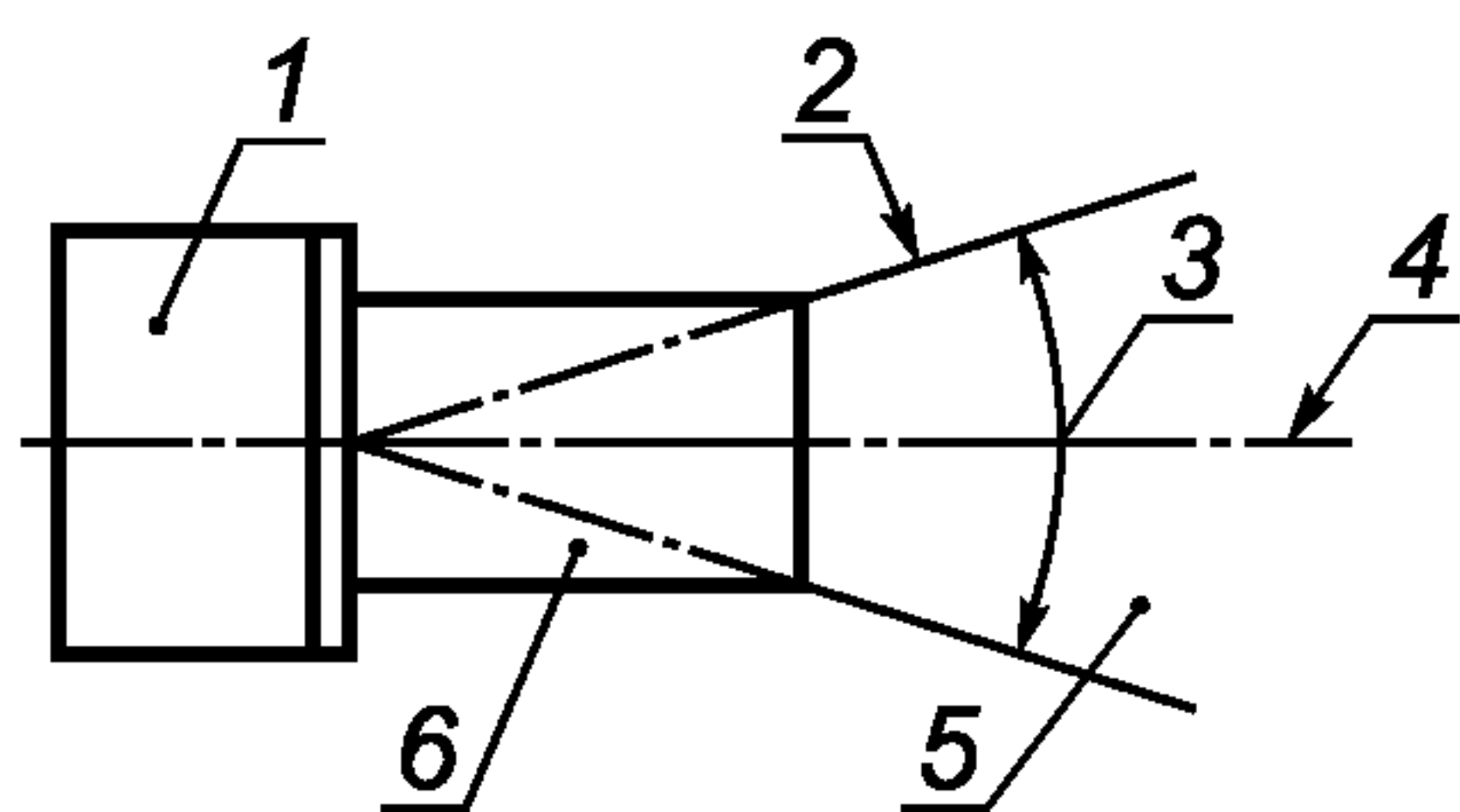
1 — прямой преобразователь (2.5.17); 2 — граница пучка (2.1.8); 3 — угол расхождения (2.3.5); 4 — ось пучка (2.1.7); 5 — дальняя зона (2.1.14); 6 — ближняя зона (2.1.18)
