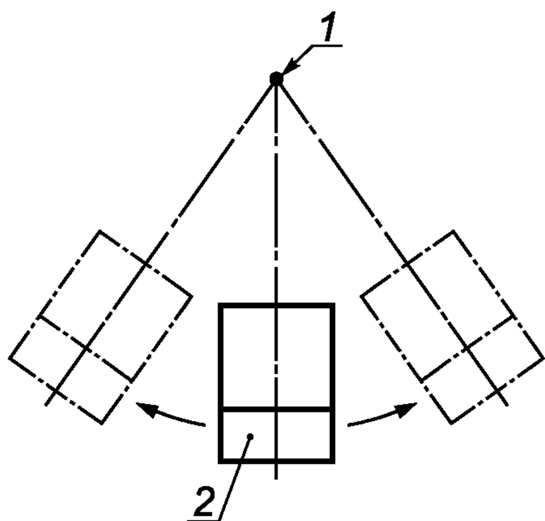
1 — несплошность (2.1.12)/дефект (2.1.15); 2 — наклонный преобразователь (2.5.1)
