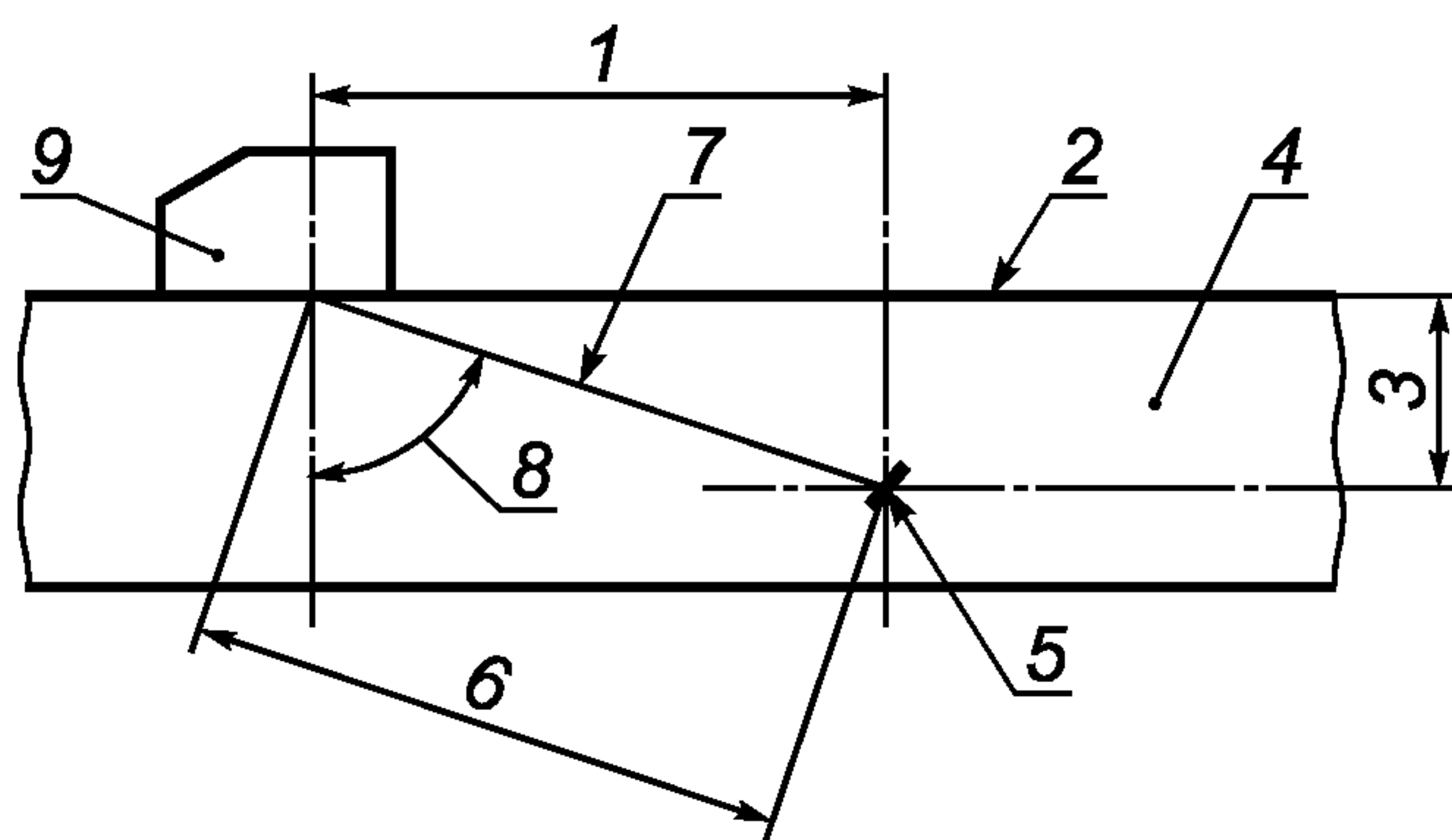
1 — проекция длины пути (2.11.2); 2 — поверхность ввода (2.9.6); 3 — глубина залегания дефекта (2.11.1); 4 — объект контроля (2.9.7); 5 — несплошность (2.1.12)/дефект (2.1.15); 6 — акустическая длина пути (2.11.4); 7 — ось пучка (2.1.7); 8 — угол преломления (2.3.3); 9 — наклонный преобразователь (2.5.1)
