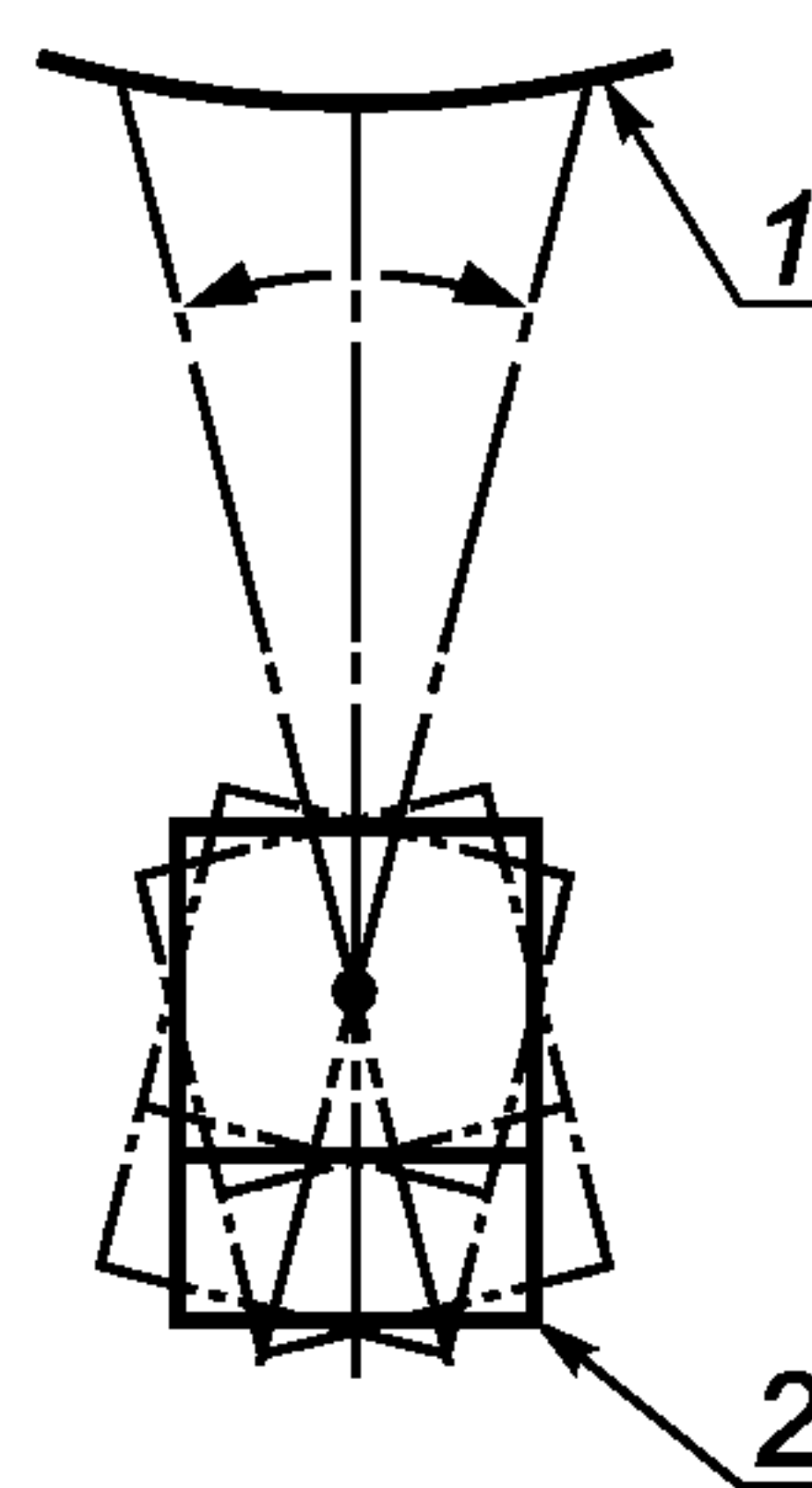
1 — несплошность (2.1.12)/дефект (2.1.15); 2 — наклонный преобразователь (2.5.1)
