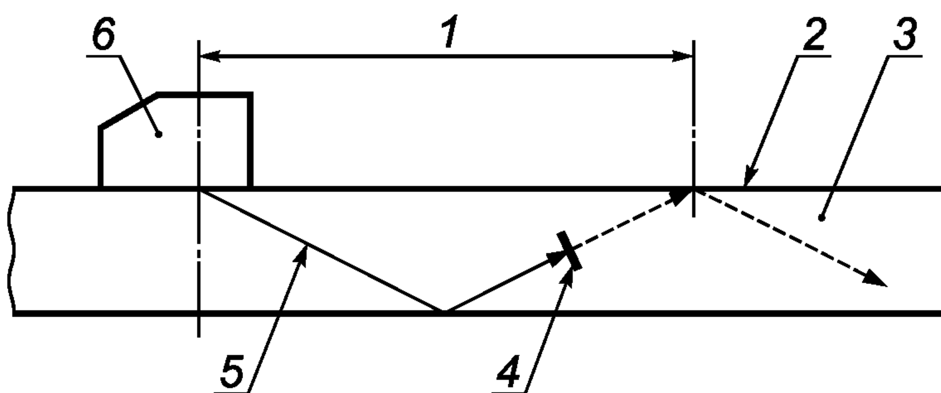
1 — расстояние однократного отражения (2.11.3); 2 — поверхность ввода (2.9.6); 3 — объект контроля (2.9.7); 4 — несплошность (2.1.12)/дефект (2.1.15); 5 — ось пучка (2.1.7); 6 — наклонный преобразователь (2.5.1)
