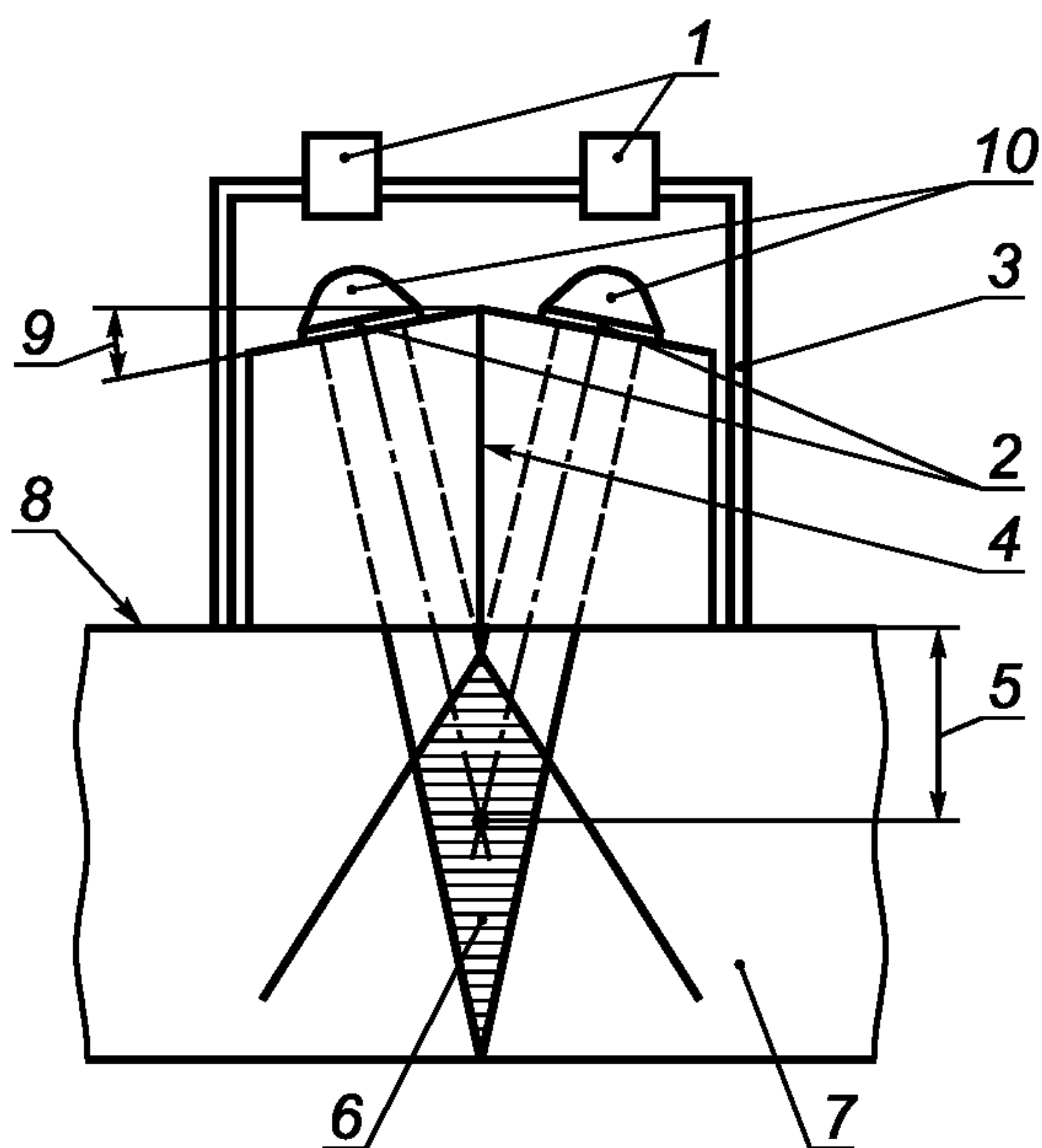
Рисунок 8 — Конструкция и ход лучей в разделяюще-совмещенном преобразователе (2.5.7)
