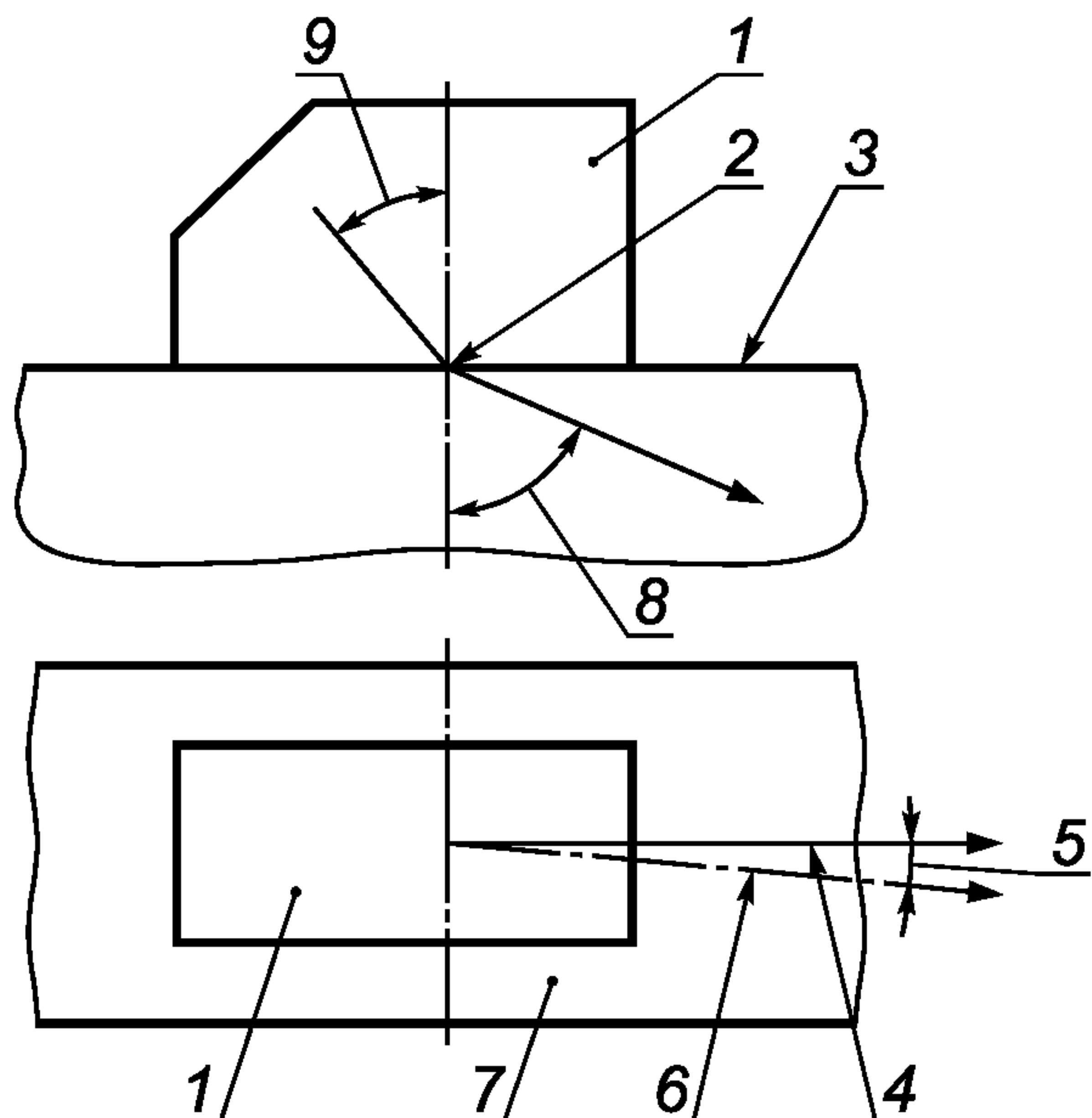
1 — наклонный преобразователь (2.5.1); 2 — точка выхода (2.5.23); 3 — поверхность ввода (2.9.6); 4 — основная ось; 5 — угол отклонения луча от оси корпуса (угол скоса) (2.5.26, 2.5.27); 6 — проекция оси пучка; 7 — объект контроля (2.9.7); 8 — угол преломления (2.3.3); 9 — угол падения (2.3.1)
