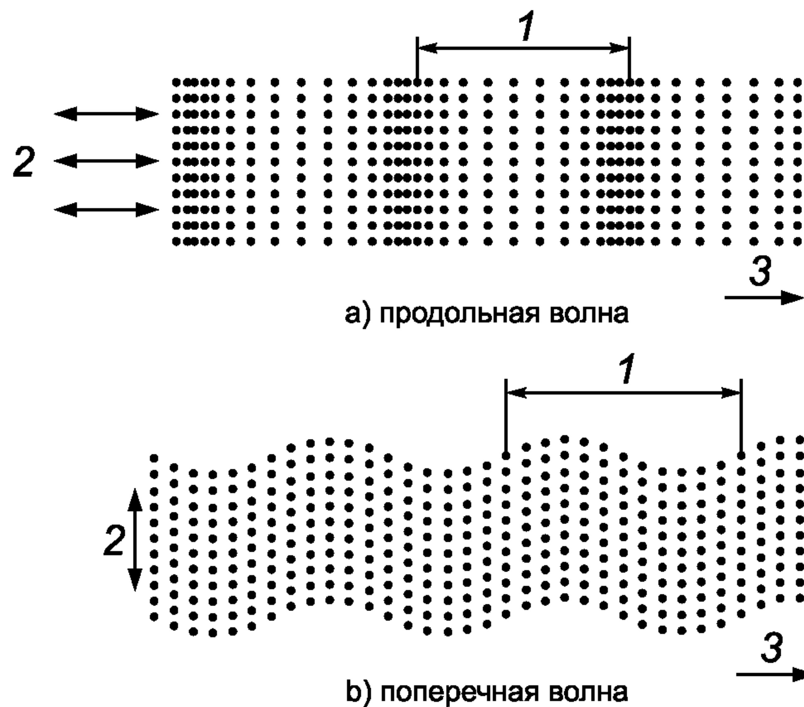
1 — длина волны (2.2.10); 2 — направление движения частиц среды; 3 — направление распространения волны
