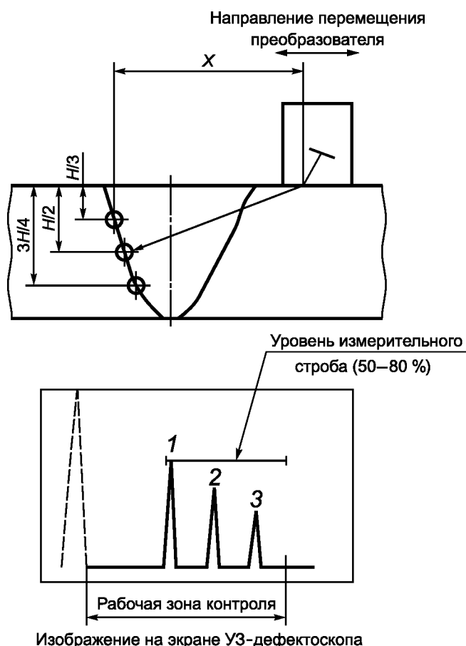
Изображение на экране УЗ-дефектоскопа
